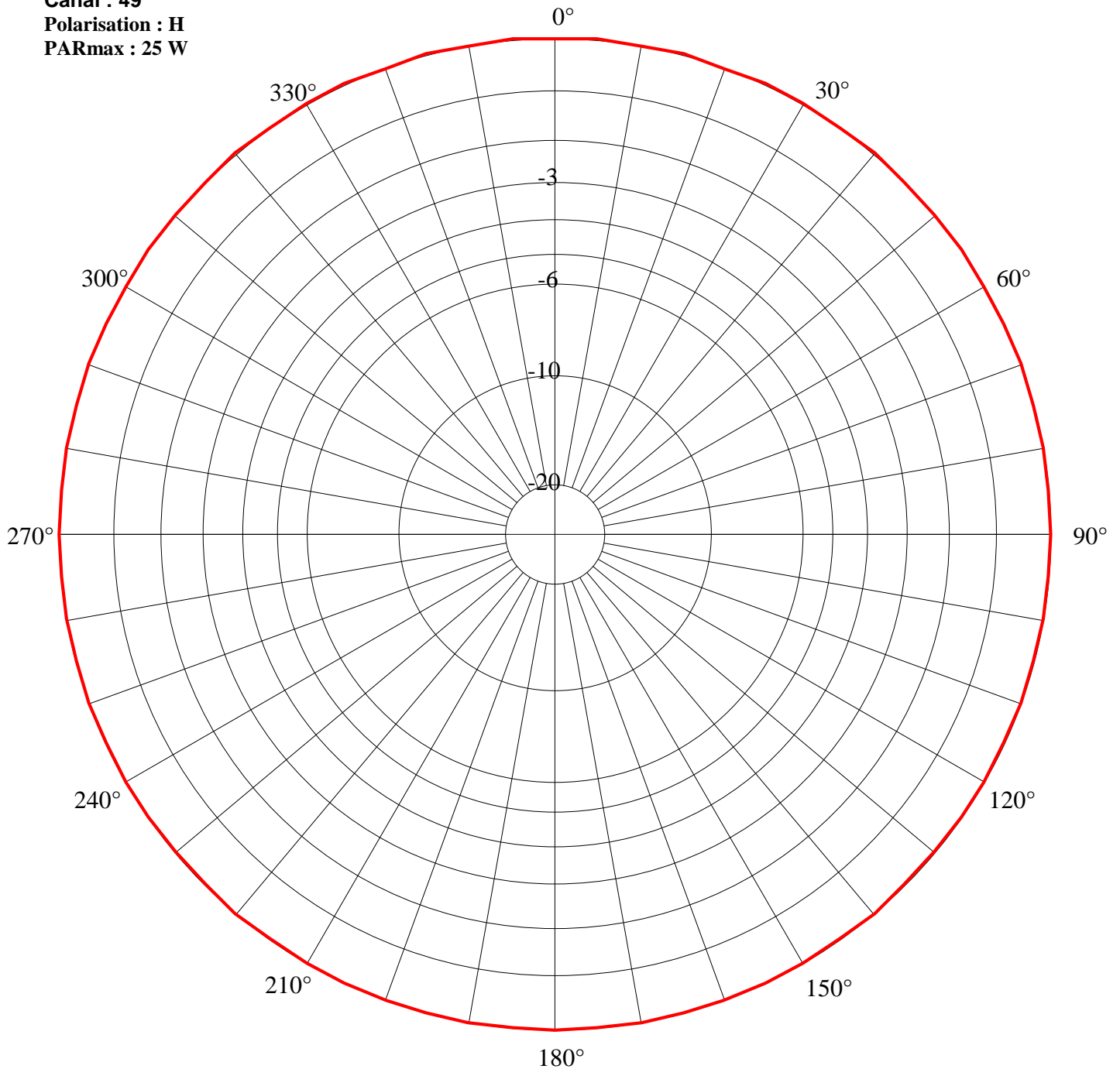
Diagramme omnidirectionnel
